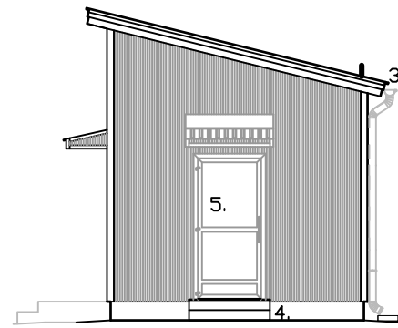
Julkisivu pohjoiseen
