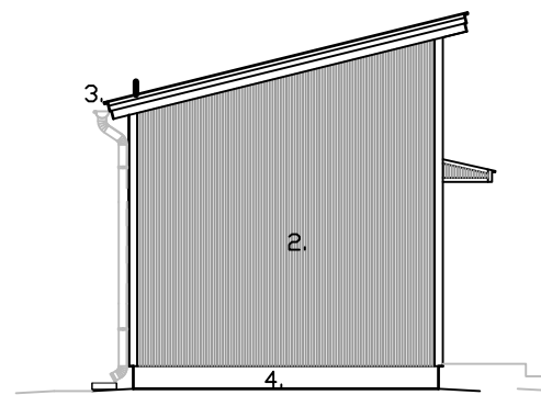
Julkisivu etelään
